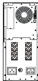
230 VAC 2200/3000 VA
